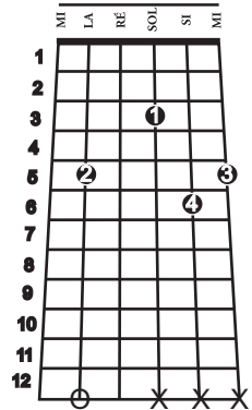
Dm(b6)
